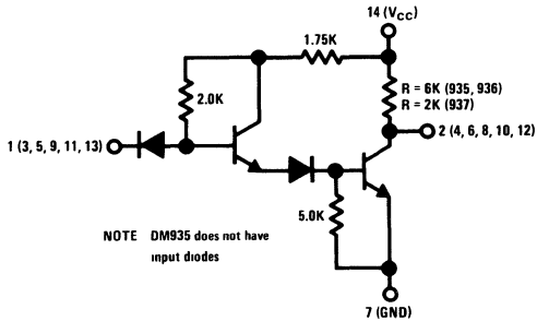
DM935/DM936/DM937
