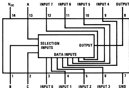
DM7210
