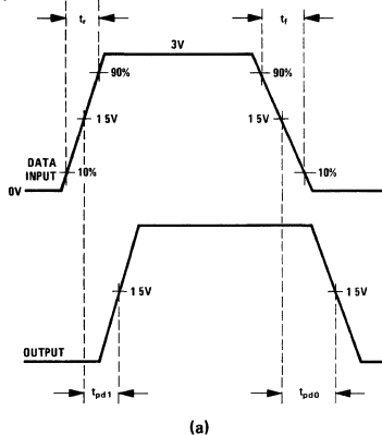
t_{pd1} & t_{pd0}
