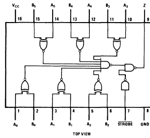
DM7160/DM8160
