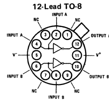
MH0026H/MH0026CH
