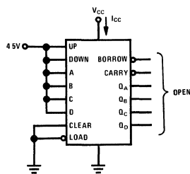
I_{CC}
