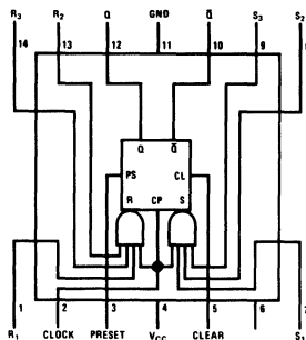
DM54L71/DM74L71
