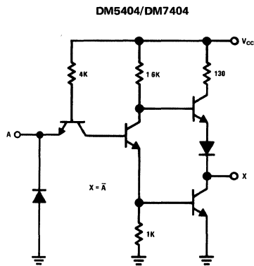
DM5404
