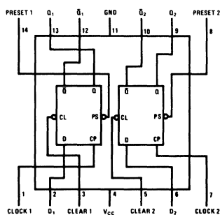
DM54L74/DM74L74
