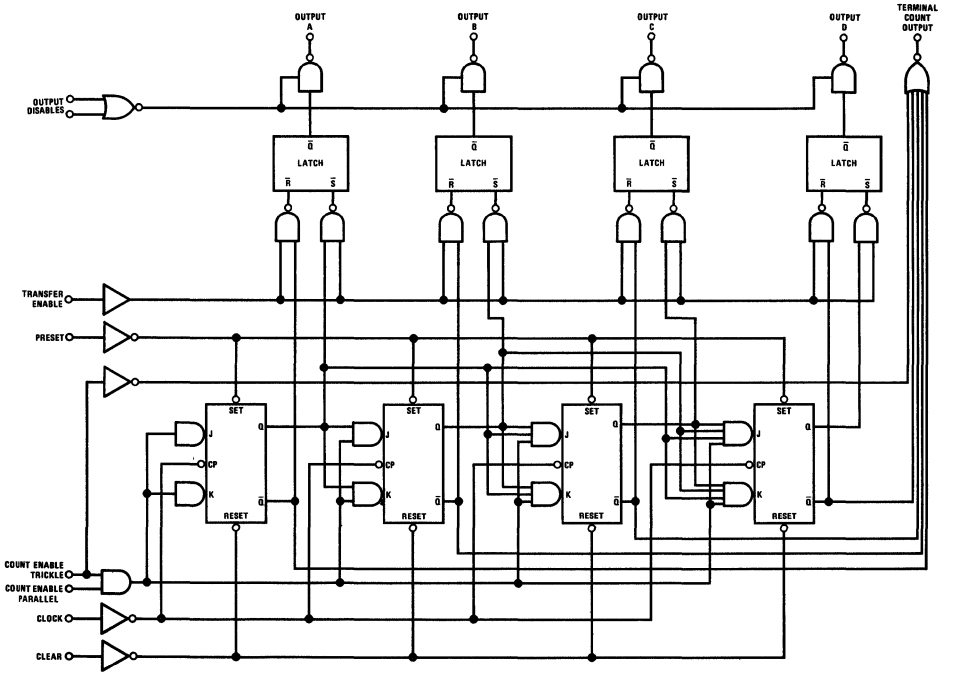
DM7554/DM8554
