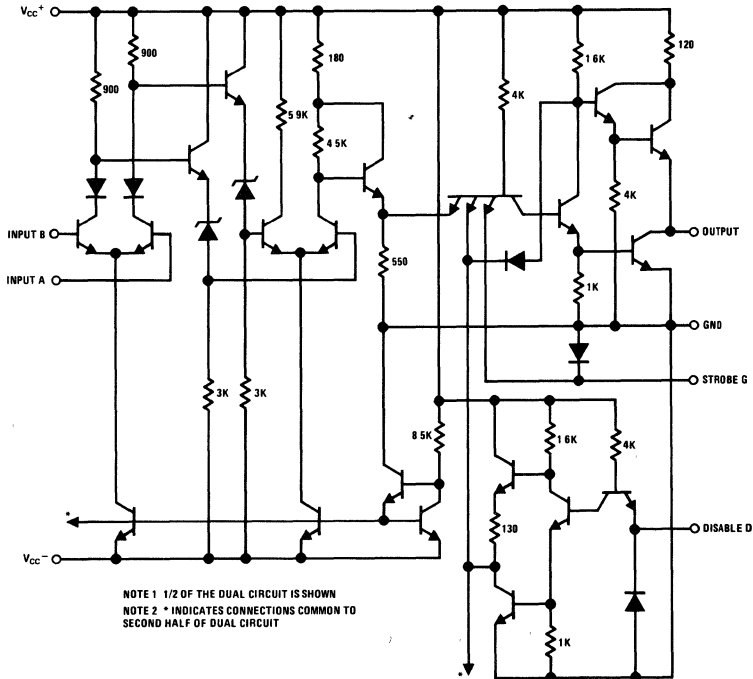
LM163/LM363, LM363A
