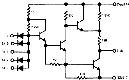
DM932
