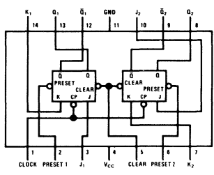
DM54L78/DM74L78
