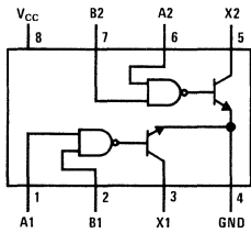
LM75461
