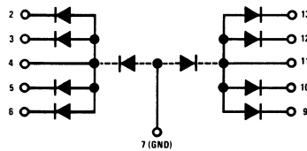
DM933
