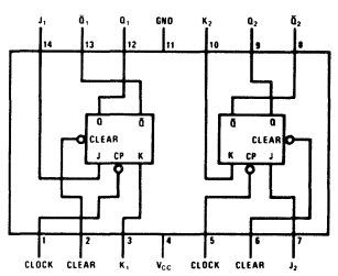
DM54L73/DM74L73
