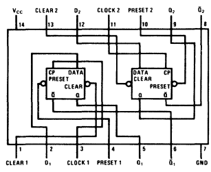
DM54L74/DM74L74
