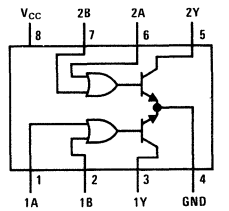
LM75464
