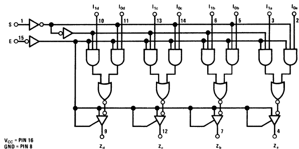
DM71L23/DM81L23
