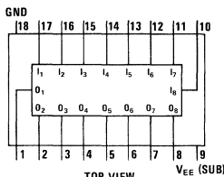
DM7887/DM8887
