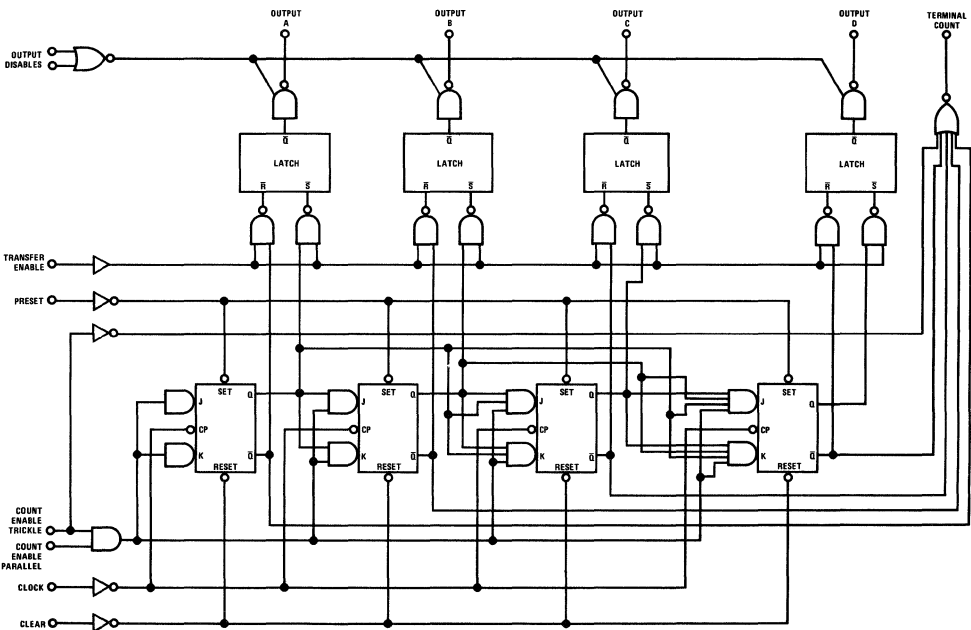
DM75L54/DM85L54
