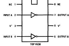
MH0026CN
