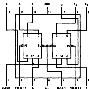
DM54L78/DM74L78
