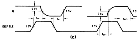
Waveform 54 (Con't)
