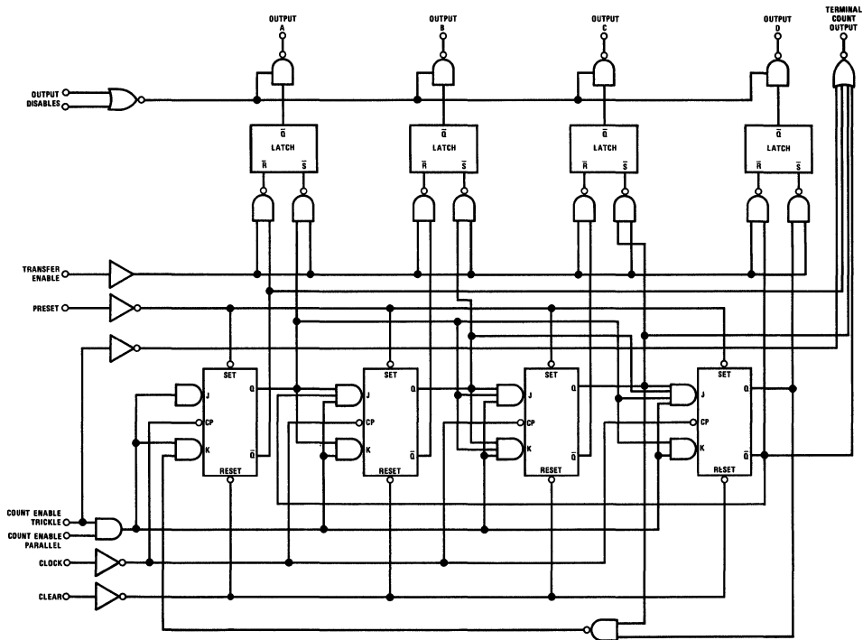
DM7554/DM8554
