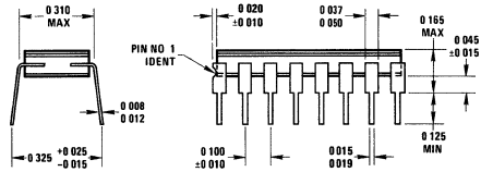
Package 9 16 Lead Cavity DIP (D)
