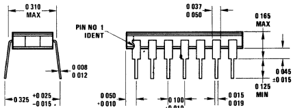
Package 8 14 Lead Cavity DIP (D)
