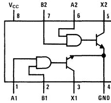
LM75462
