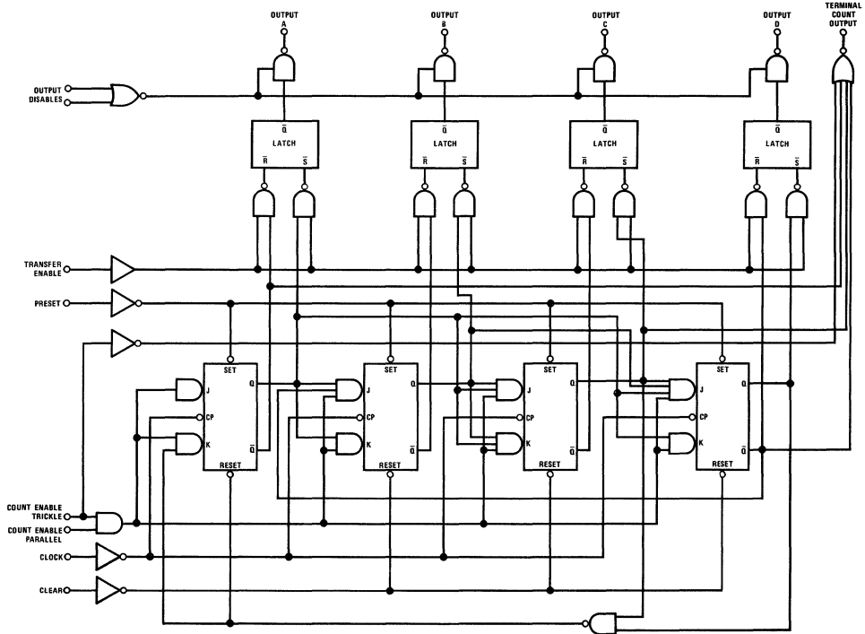
DM75L54/DM85L54
