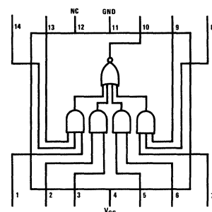
DM54L54/DM74L54
