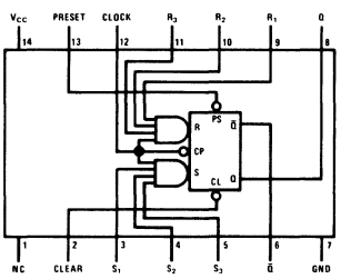
DM54L71/DM74L71
