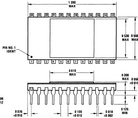
Package 10 24 Lead Cavity DIP (D)
