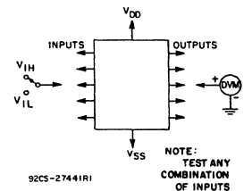
Fig. 17 – Input-voltage test circuit.
