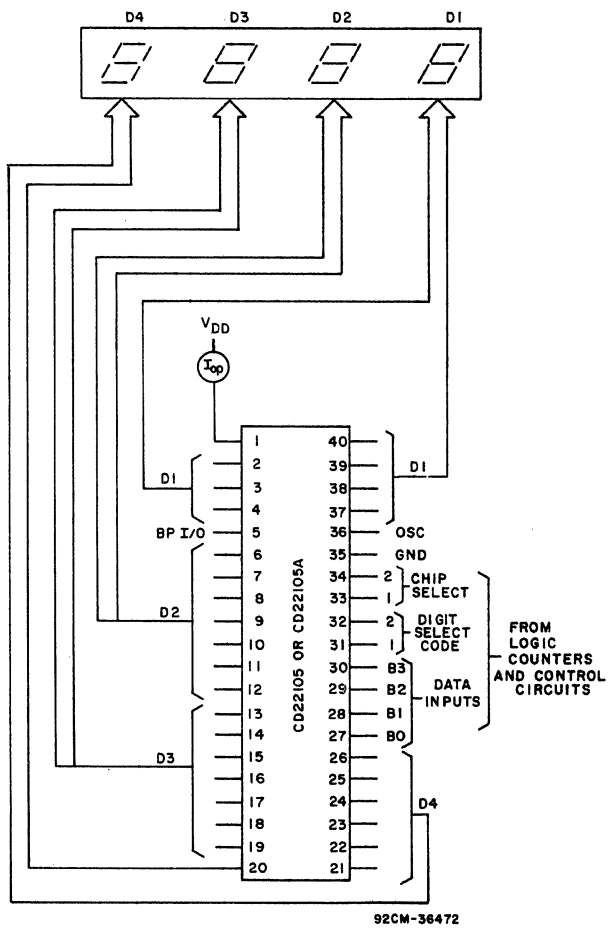
Fig. 5 - Test circuit.
