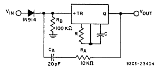
Fig. 22 - Input-pulse stretcher circuit.
