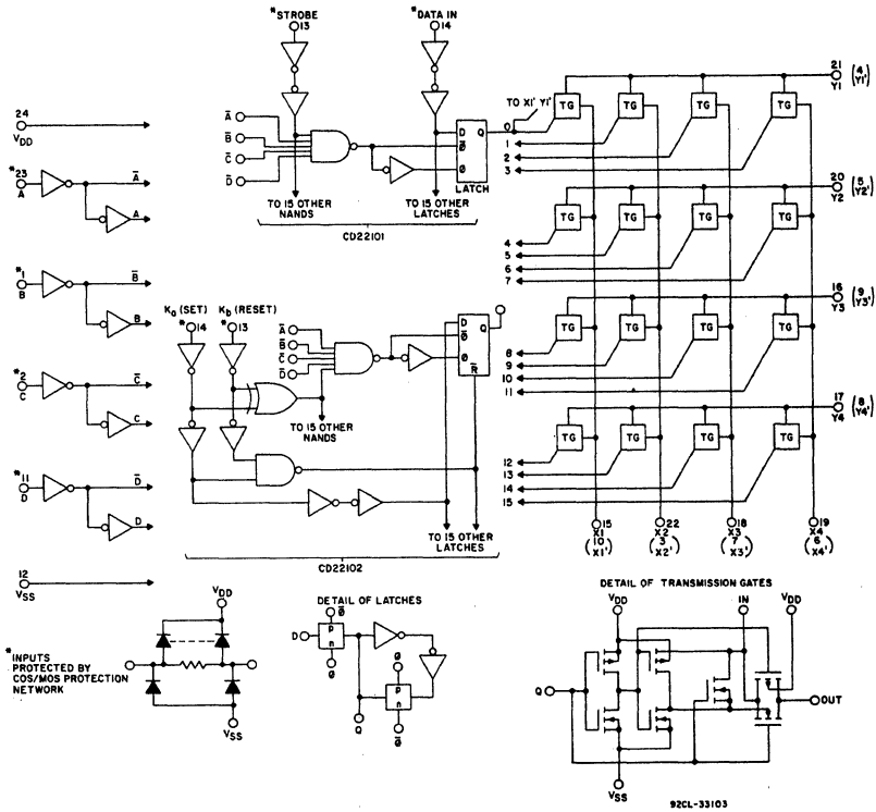
Fig. 2 - Logic diagram.
