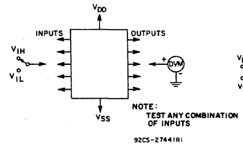
Fig. 10 – Input voltage.
