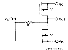
Fig. 5— COS/MOS amplifier.
