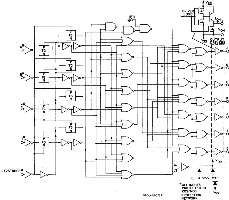
Fig. 8 - Logic diagram.
