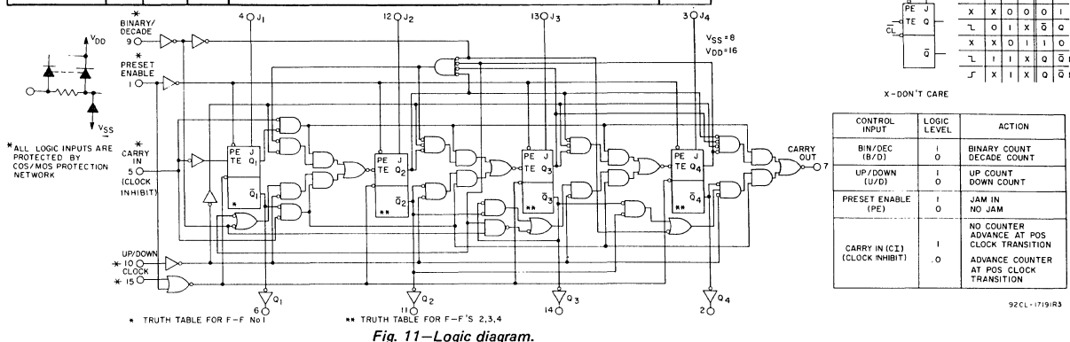
Fig. 11—Logic diagram.
