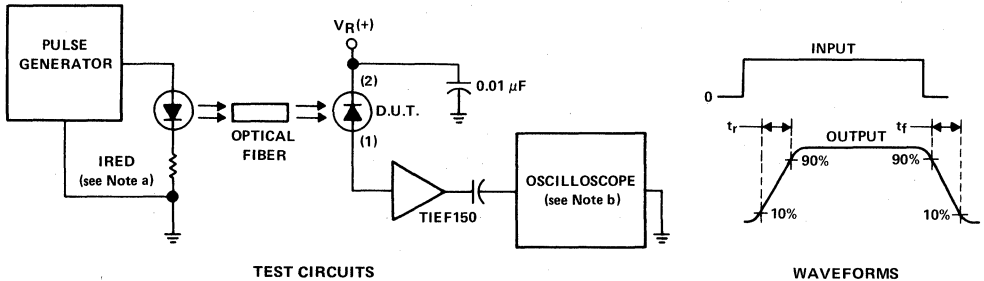
TEST CIRCUITS
