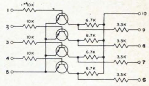
UD-4024 BUFFER AMPLIFIER
