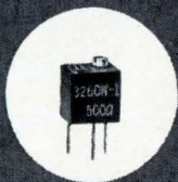
New TRIMPOT® Potentiometer Model 3260W ACTUAL SIZE
